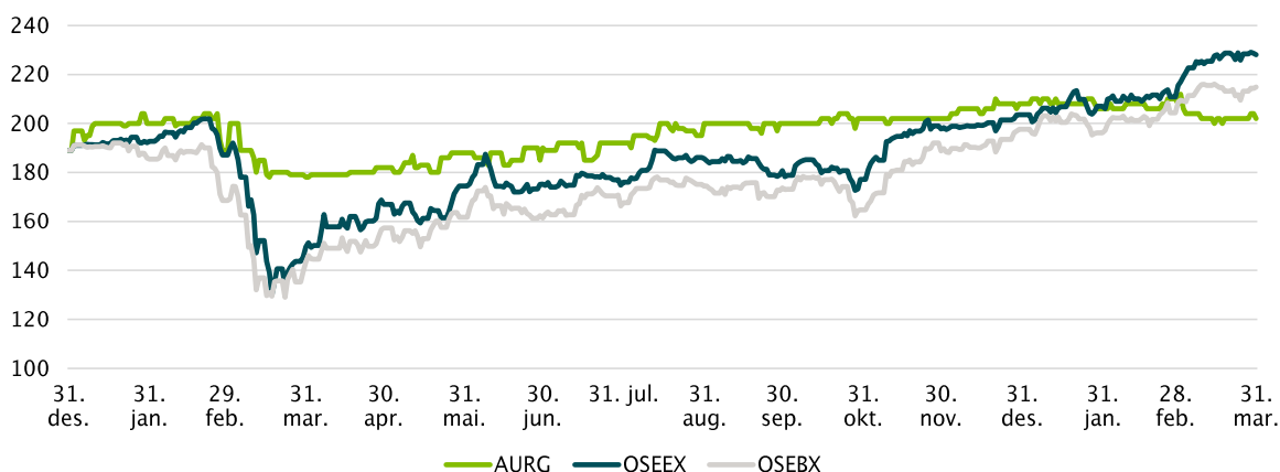
Kursutvikling siste 15 måneder
